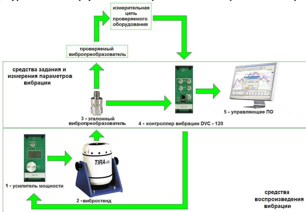
Рисунок 1 – Структурная схема виброустановки поверочной DVC-500
