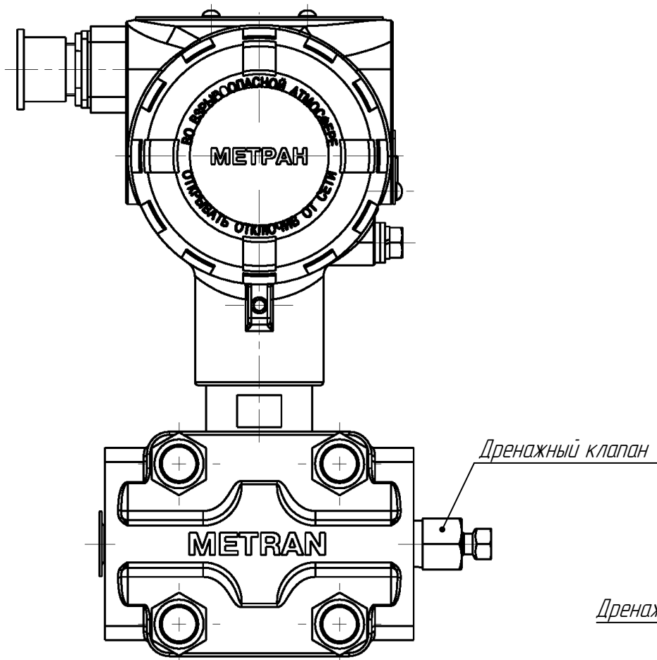
Рисунок Ж.15 – Датчики модели 150CD, 150CG. Варианты расположения дренажных клапанов
