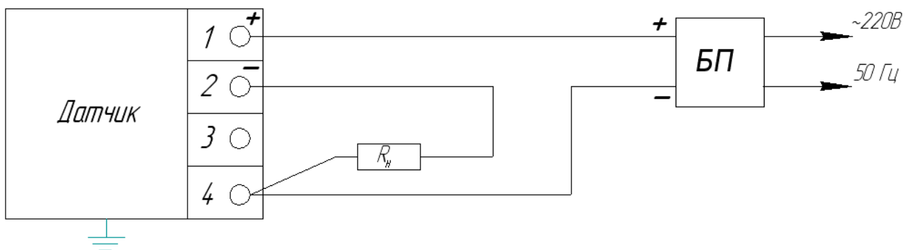
Рисунок Г.2.2 – Выходной сигнал 4-20 мА (вариант соединения)
