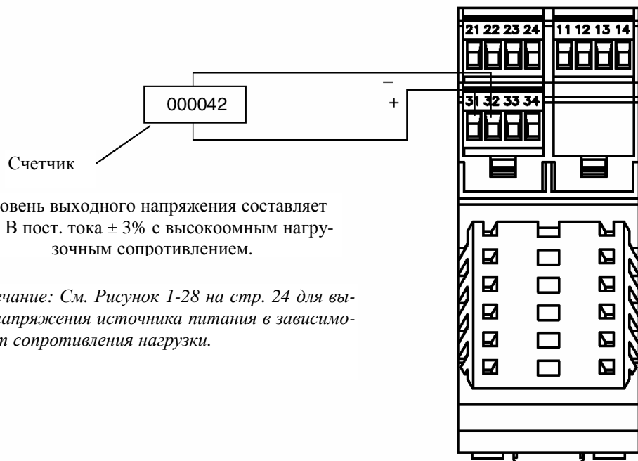
Рисунок 1-21. Подключение частотного выхода для клемм 31 & 32 с внутренним питанием
