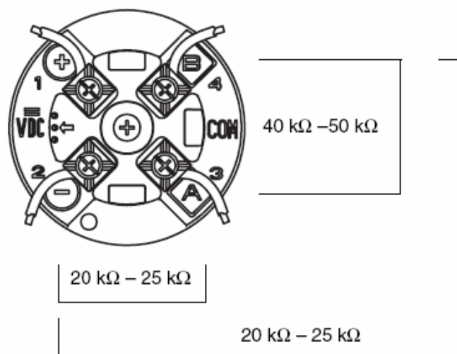
Рисунок 10-1 Тестирование сопротивлений базового процессора
