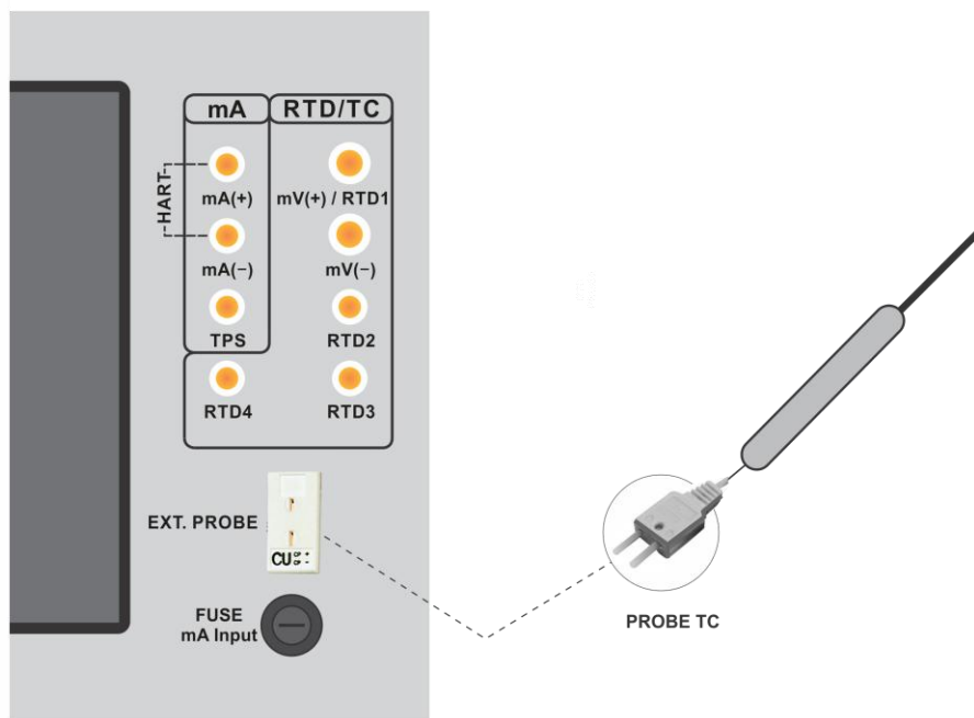
Рис. 12 - Подключение эталонного датчика в качестве внешнего эталона
