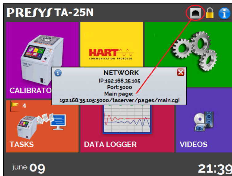
Рис. 34 - IP-адрес
