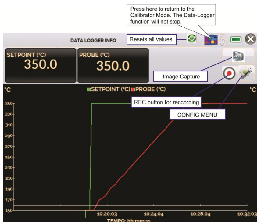
Рис. 34 - Регистратор данных
