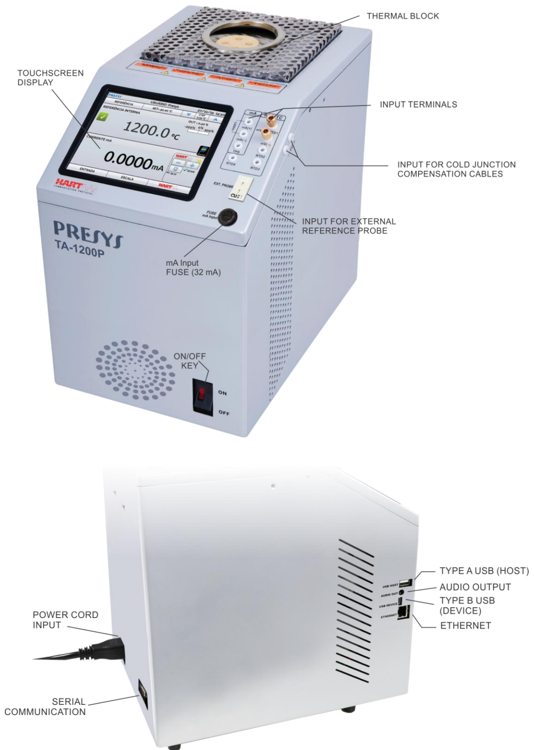
Рис. 05 - Внешний вид калибратора температуры
