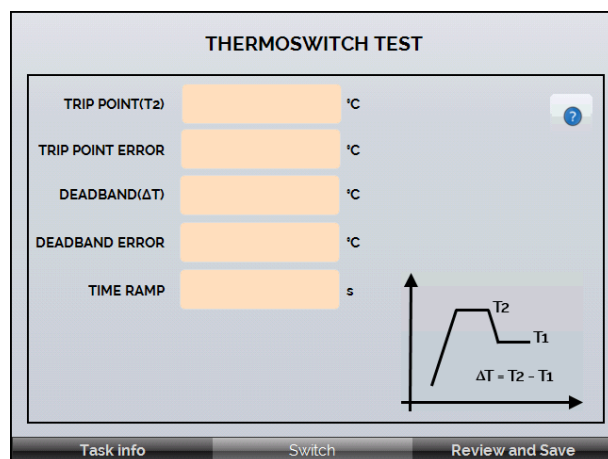
Fig 29 – Параметры задания для реле температуры (SWITCH)
