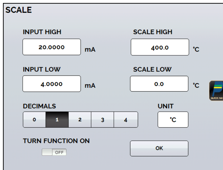
Рис. 20 - Настройка функции Scale (Шкала)
