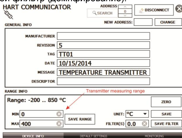
Рис. 23 - Калибровка диапазона измерений измерительного преобразователя с протоколом HART®
