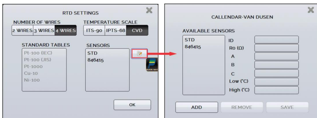
Рис. 11 – Настройки для входного сигнала RTD (ТС)
