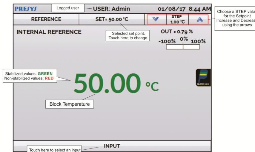
Рис. 05 – Режим калибратора
