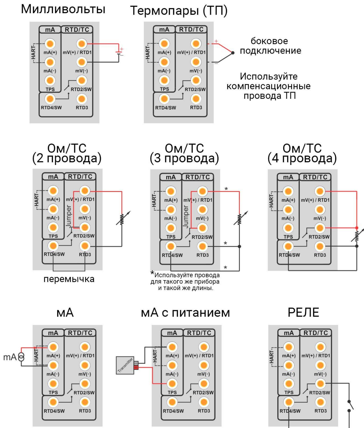
Рис. 14 – Внешние подключения
