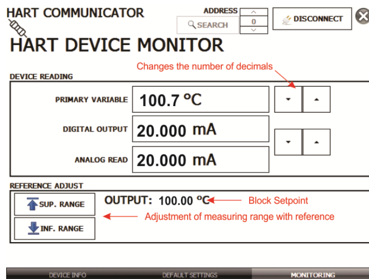
Рис. 22 – Калибровка диапазона измерений измерительного преобразователя с протоколом HART® при помощи эталона
