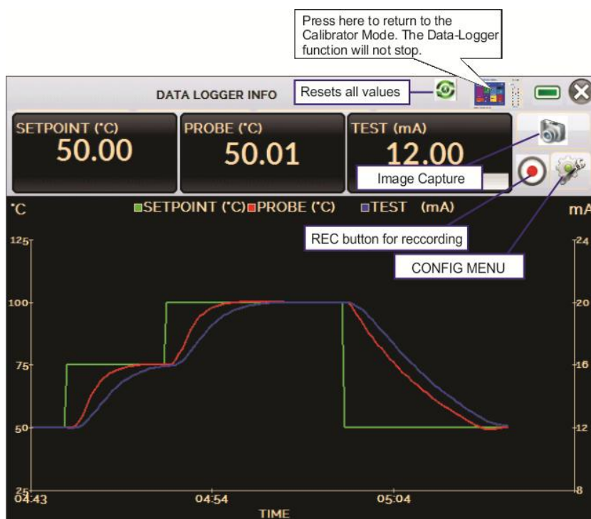
Рис. 31 – Регистратор данных
