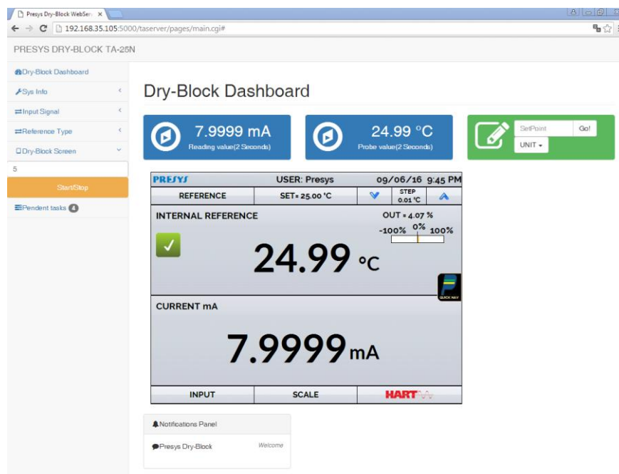
Рис. 33 – Интернет-сервер калибратора ТА
