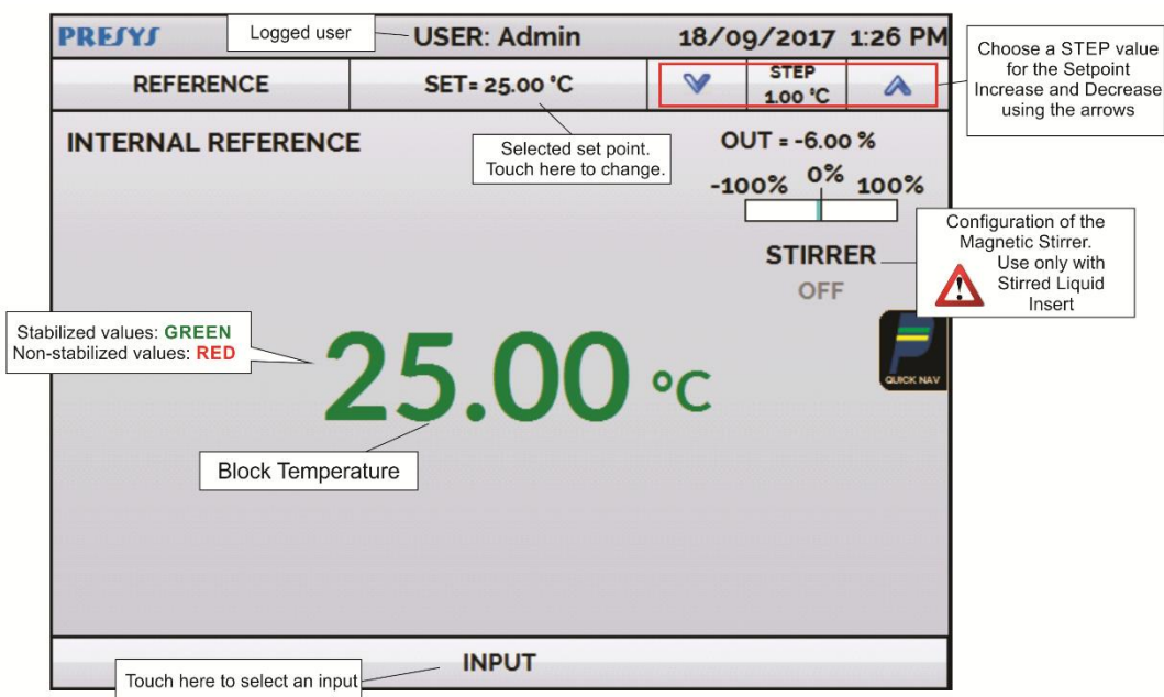
Рис. 06 - Режим калибратора
