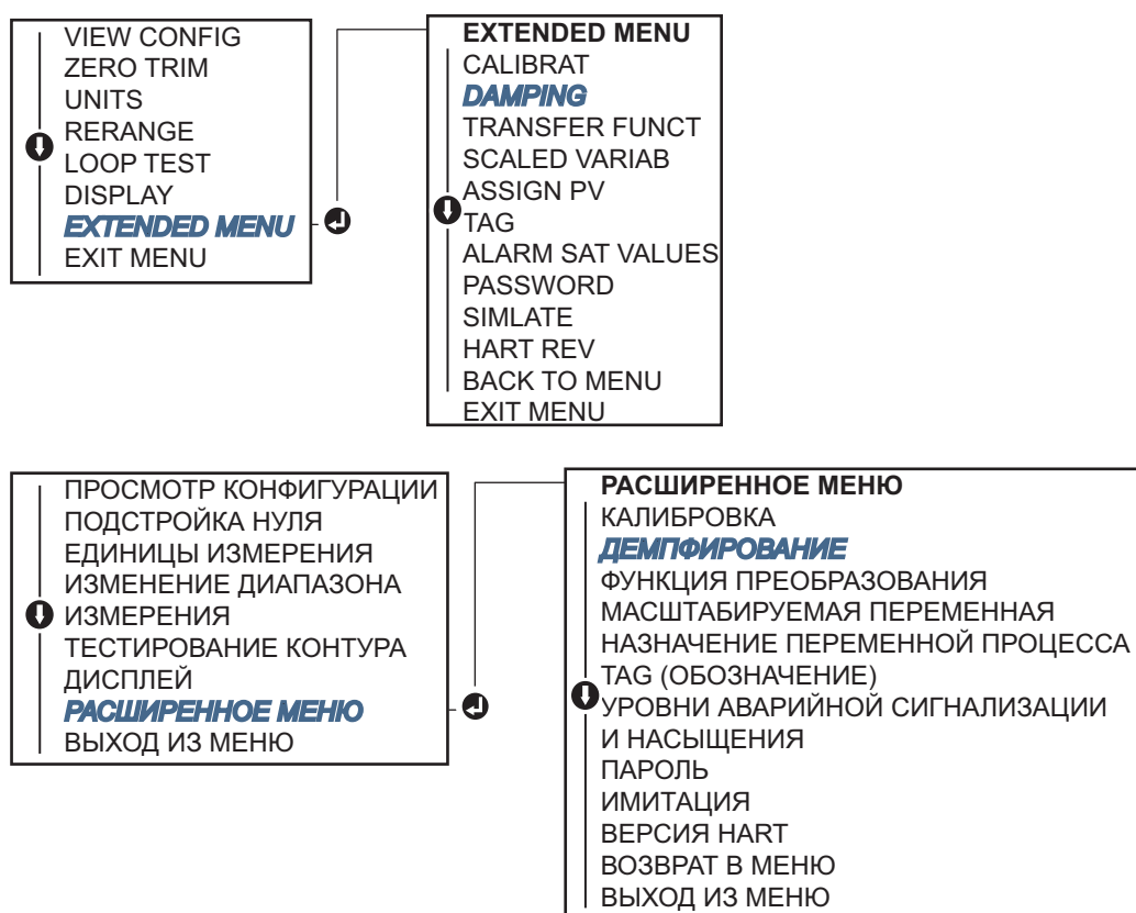
Рисунок 2-10. Задание времени демпфирования с помощью локального интерфейса оператора
