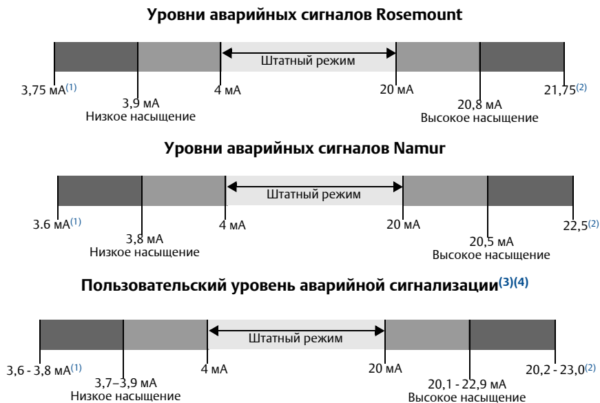
Рисунок 7-1. Уровни сигнализации
