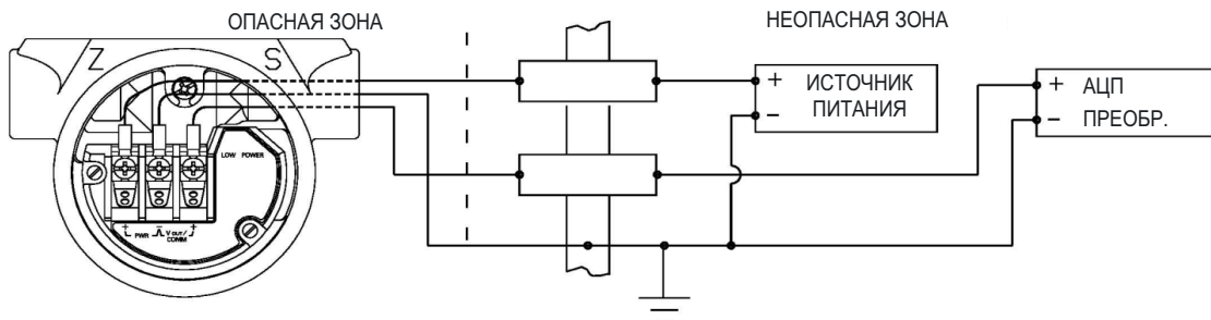
ПРИНЦИПИАЛЬНАЯ СХЕМА 4 ДВА ОДНОКАНАЛЬНЫХ БАРЬЕРА (ДЛЯ ПРИМЕНЕНИЯ ТОЛЬКО С БАРЬЕРАМИ, ОДОБРЕННЫМИ В ЭТОЙ КОНФИГУРАЦИИ)
