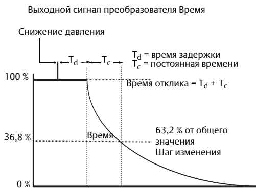
Рисунок А-1. Номинальное время отклика преобразователя по протоколу HART
