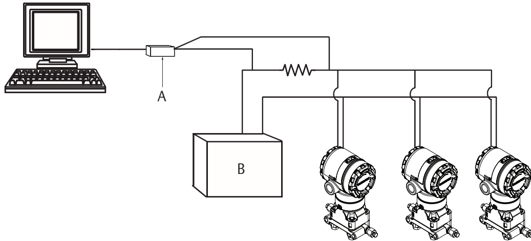
Рисунок 2-19. Стандартная многоточечная сеть
