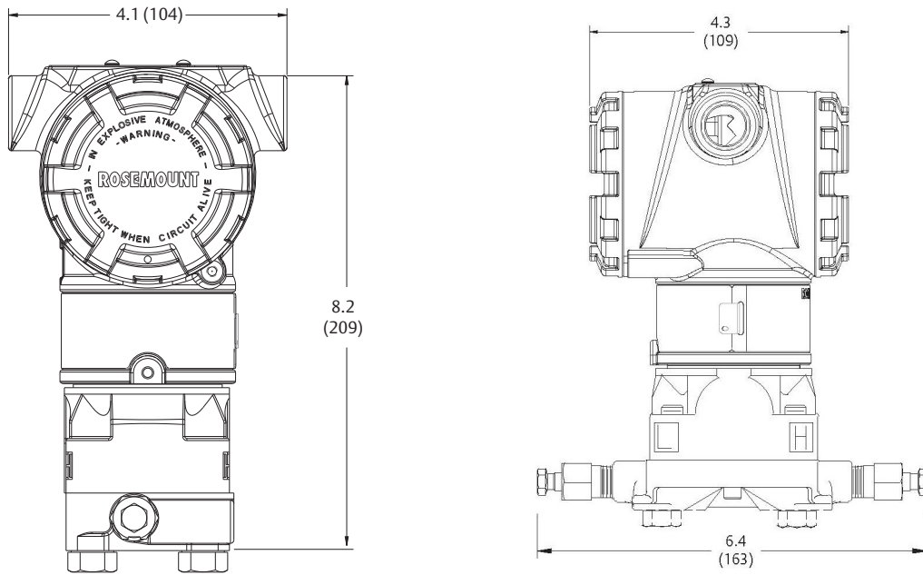
Рисунок А-3. Расширенный преобразователь 3051С с фланцем Sorlapar
