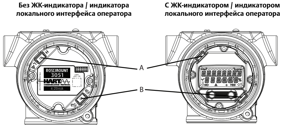
Рис. 4-2. Электронная плата
