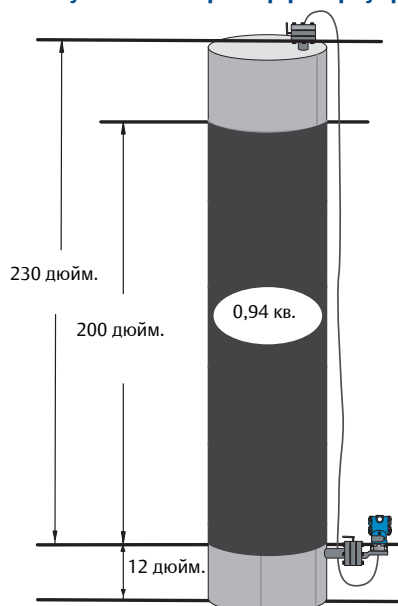
Рисунок 2-14. Пример резервуара
