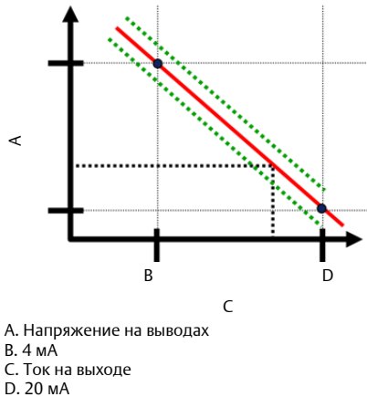
Рисунок 2-16. Основная рабочая зона
