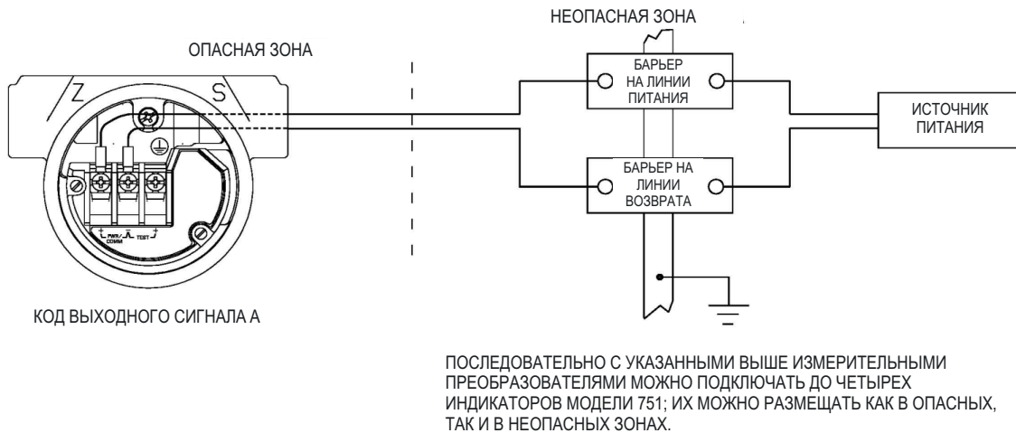
ПРИНЦИПИАЛЬНАЯ СХЕМА 2 БАРЬЕРЫ ПО ПИТАНИЮ И ОБРАТНЫЕ БАРЬЕРЫ (ДЛЯ ПРИМЕНЕНИЯ ТОЛЬКО С БАРЬЕРАМИ, ОДОБРЕННЫМИ В ЭТОЙ КОНФИГУРАЦИИ)
