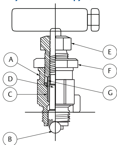
Рисунок 3-13. Конструкция вентиля
