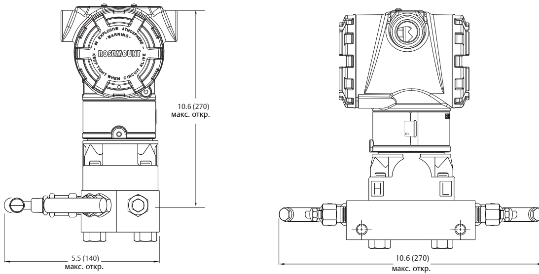
Рисунок А-4. Преобразователь 3051С с фланцем Sorlapar со встраиваемым трехвентильным клапанным блоком Rosemount 305
